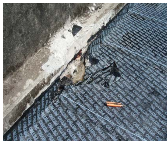
防水膜遇落水頭收頭
