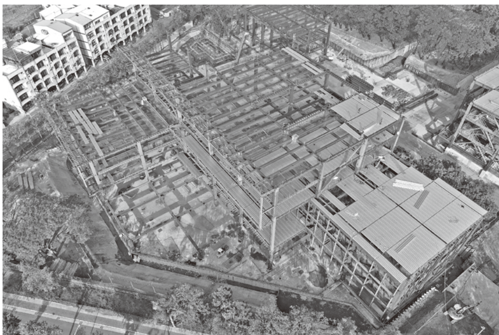
圖 28 國圖南部分館暨國家聯合典藏中心結構空拍圖
