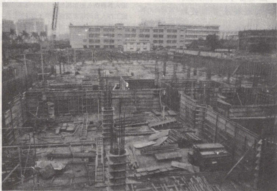
地下室一層柱、牆模板工程
