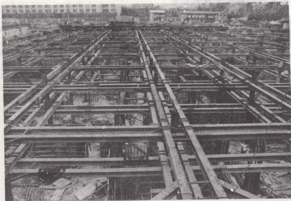
地下室一層支撐工程
