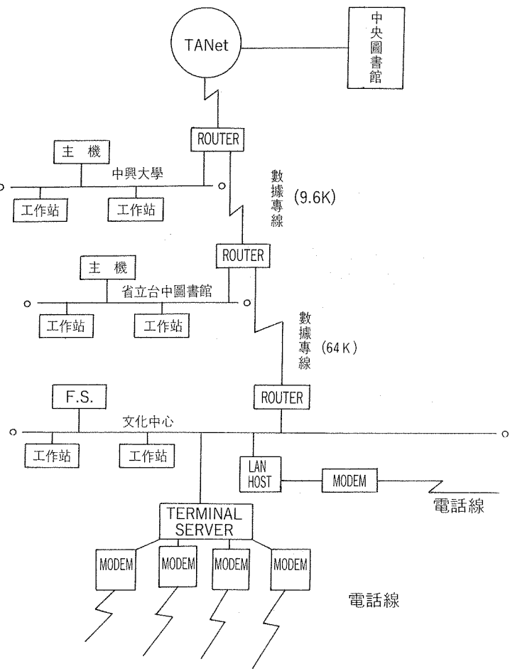
彰化縣立文化中心圖書館連線架構圖
